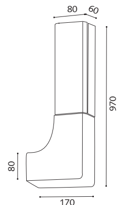
Serbatoio Extralarge Volume di lavoro 19 cm 3 Attacchi di aspirazione su entrambi i lati del serbatoio
